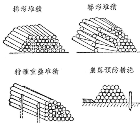
圖 14：木材堆積法
